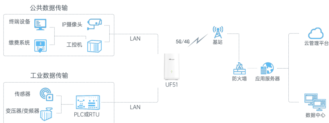
图 1.1 概述-1
