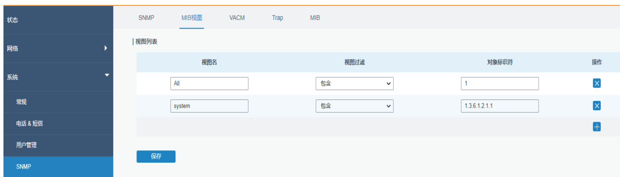
图 3.3.4.2 MIB 视图-75
