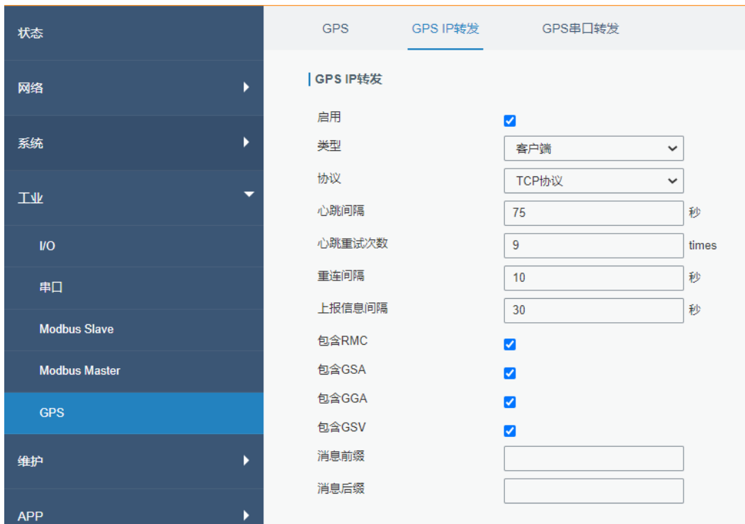
图 3.4.5.2 GPS IP 转发-97
