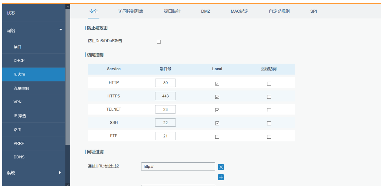
图 3.2.3.1 安全-25
