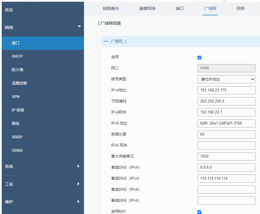
图 3.2.1.4 广域网-14
